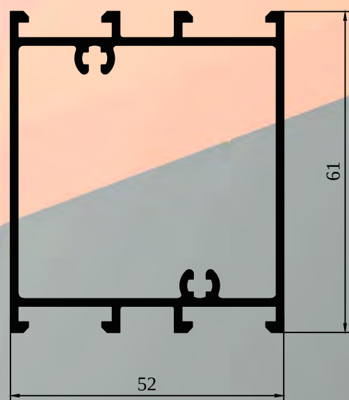
ALX-2218 TRAVESAÑO HOJA PUERTA REVATIR
