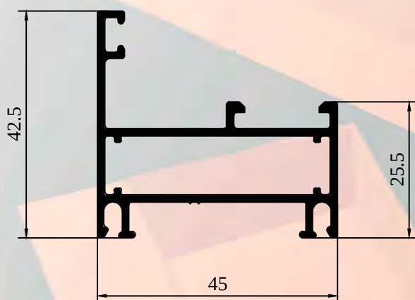
ALX-2216 MARCO VENTANA DE ABRIR
