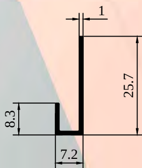
ALX-J Peso : 0.105 Kg/m
