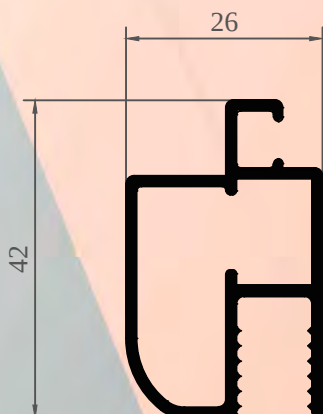
ALX-6038 BASTIDOR MOSQUITERO
