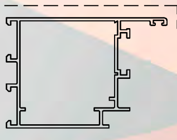
ALX-2214 JAMBA Y CABEZAL HOJA DE PUERTA
