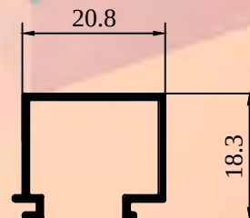
ALX-1108 CONTRAVIDRIO UNIVERSAL Peso : 0.180 Kg/m
