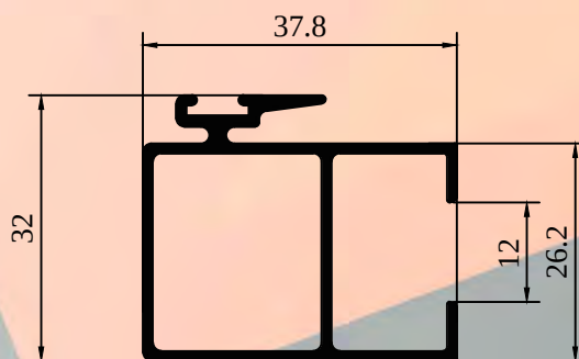
ALX-2207 PARANTE CENTRAL PUERTA Y VENT. CORREDIZA VID. SIMPLE
