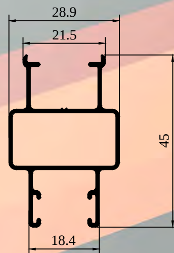
ALX-1003 PARANTE LATERAL Peso : 0.400 Kg/m
