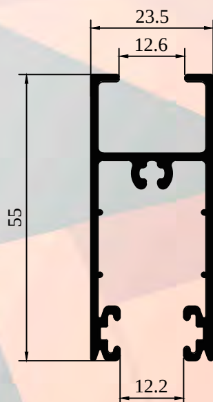
ALX-2204 ZÓCALO Y CABEZAL DE HOJA
