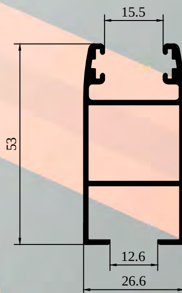
ALX-2203 PARANTE LATERAL DE HOJA
