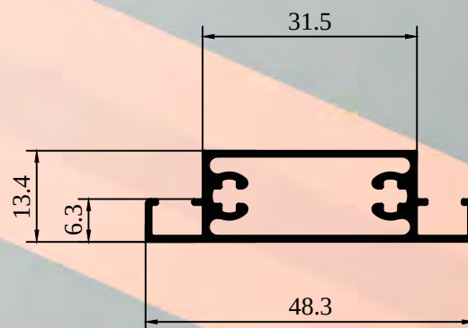
ALX-1990 TRAVESAÑO MOSQUITERO
