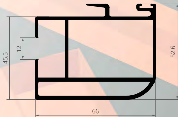
ALX-6035 PARANTE CENTRAL
