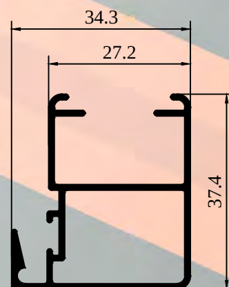
ALX-3054 PARANTE CENTRAL HOJA VENTANA CORREDIZA Peso : 0.694 Kg/m
