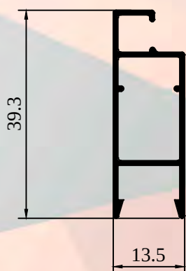
ALX-1905 MOSQUITERO CORREDIZO
