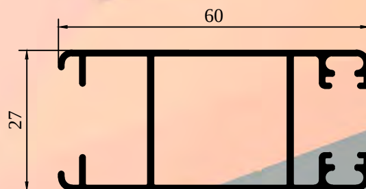
ALX-3053 PARANTE LATERAL Peso : 0.645 Kg/m
