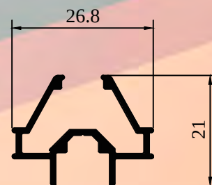
ALX-1774 BASTIDOR VIDRIO REPARTIDO
