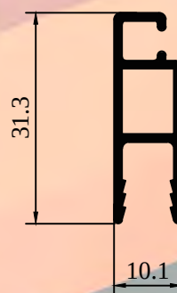
ALX-1110 MOSQUITERO LIVIANO
