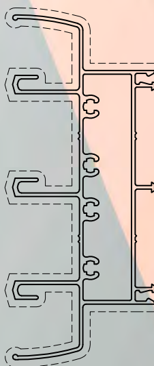
ALX-2240 UMBRAL Y DINTEL MARCO DE 3 GUÍAS
