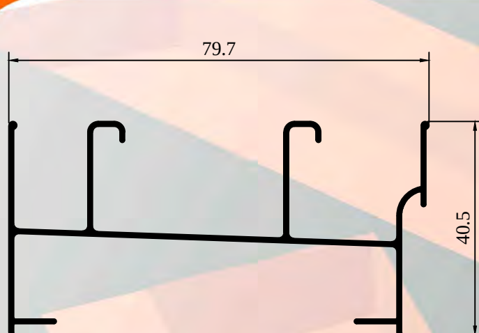
ALX-1001 MARCO LIVIANO Peso : 0.575 Kg/m
