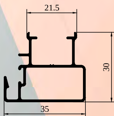
ALX-1004 HOJA LATERAL Peso : 0.364 Kg/m
