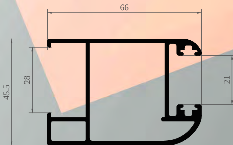
ALX-6071 PARANTE LATERAL DVH Peso : 1.291 Kg/m
