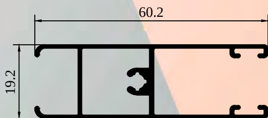
ALX-3052 ZOCALO 90° Peso : 0.496 Kg/m
